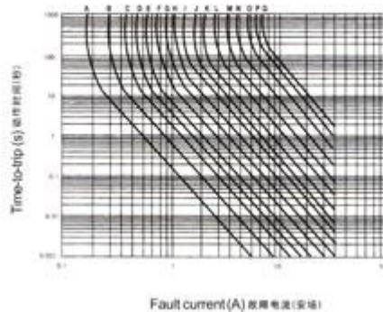
WH60系列 25°C 时典型动作时间曲线
