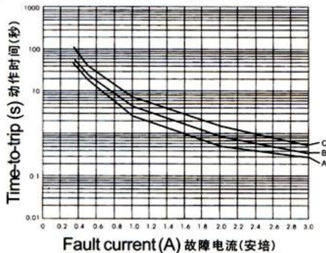
WH600系列 25°C 时典型动作时间曲线
