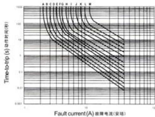
WH30系列 25°C 时典型动作时间曲线
