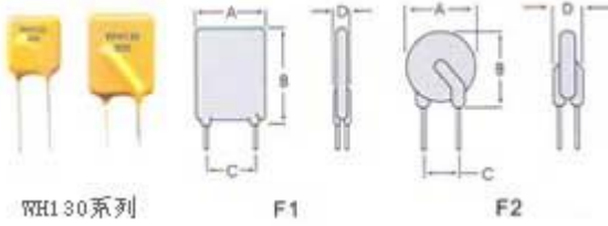
WH130系列 电器特征与产品尺寸
